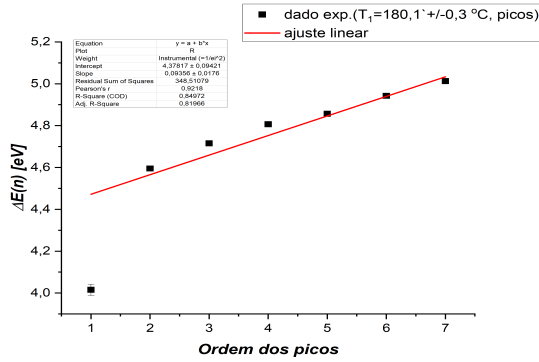
Fig. 2 Ajuste linear da diferença de energia entre dois picos consecutivos pela ordem dos picos referente a primeira aquisição.
