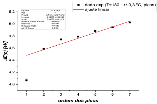
Fig. 4 Ajuste linear da diferença de energia entre dois picos consecutivos pela ordem dos picos referente a segunda aquisição.
