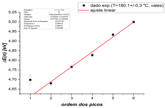
Fig. 5 Ajuste linear da diferença de energia entre dois vales consecutivos pela ordem dos picos referente a segunda aquisição.
