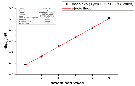
Fig. 3 Ajuste linear da diferença de energia entre dois vales consecutivos pela ordem dos picos referente a primeira aquisição.
