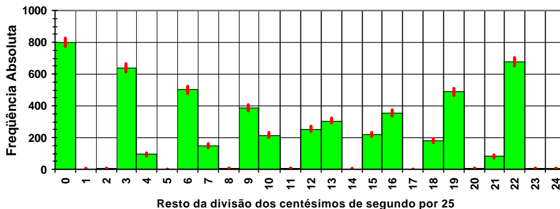
Figura 4 – Distribuição de ocorrências de 5 391 resultados de cronometragens apenas dos cronômetros que apresentam o comportamento analisado. Os tempos amostrados variam entre ~0,5 e ~30 s.
